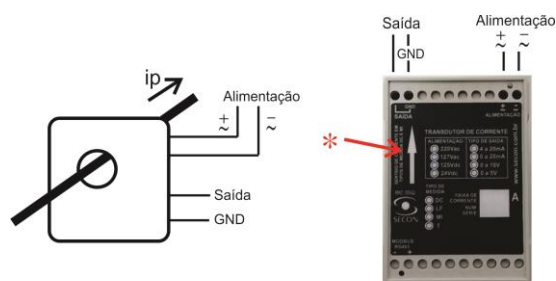
Encapsulamento Tipo1
