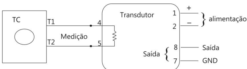
Conexão TC (Transformador de Corrente)
