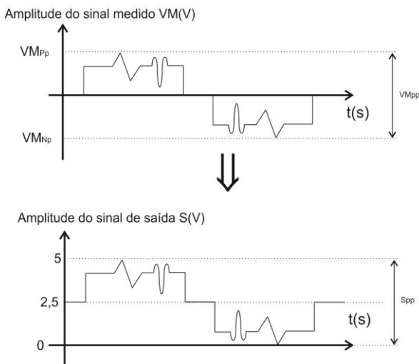
Transdutores com saída (0-5)Vdc
