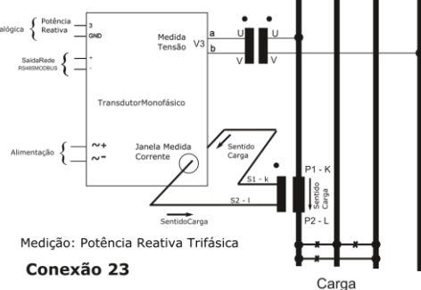
Cargas Equilibradas (1 elementos 4 fios) Modelo Janelado com TC e TP
