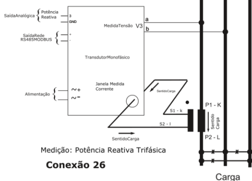
Cargas Equilibradas (1 elementos 3 fios) 1 fase simulada - 1FS Modelo Janelado com TC
