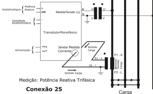
Cargas Equilibradas (1 elementos 4 fios) Modelo Janelado com TC, TP e Aterramento
