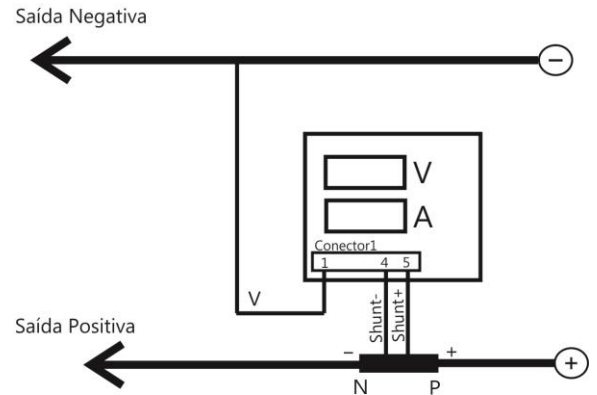
SHUNT EM SÉRIE COM A SAÍDA POSITIVA
