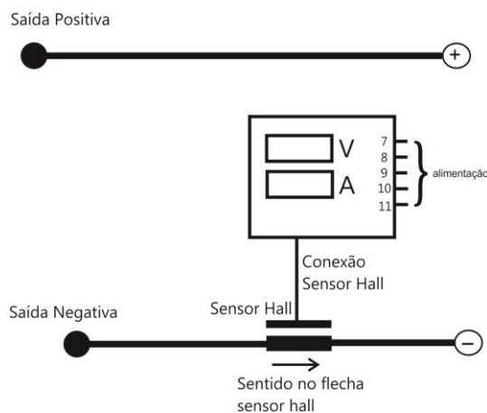
SENSOR HALL EM SÉRIE COM A SAÍDA NEGATIVA
