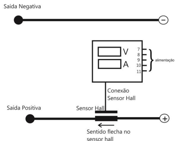
SENSOR HALL EM SÉRIE COM A SAÍDA POSITIVA
