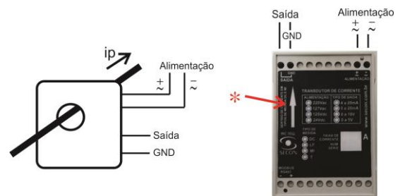
Encapsulamento Tipo1
