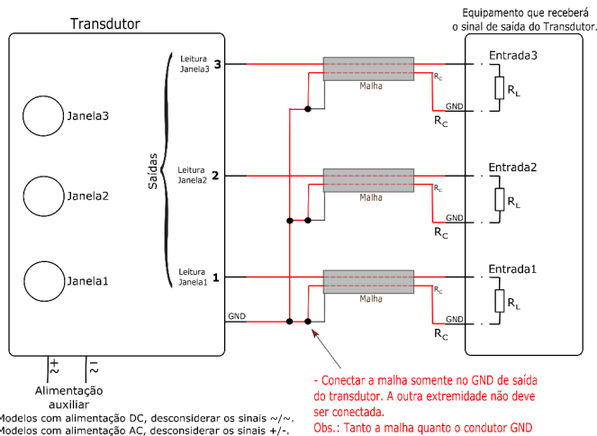
(Conexão com cabo blindado)
