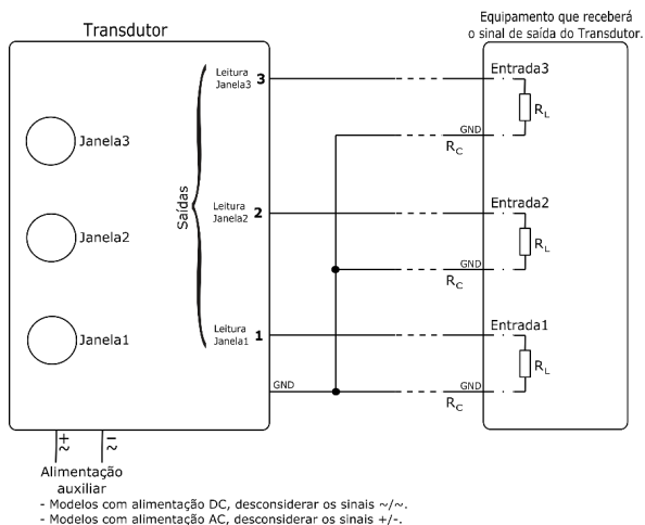
(Conexão sem cabo blindado)
